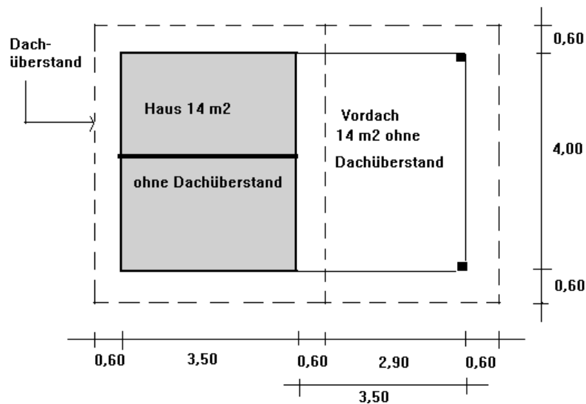
Detailzeichnung Pergola/Vordach im Wochenendgarten
