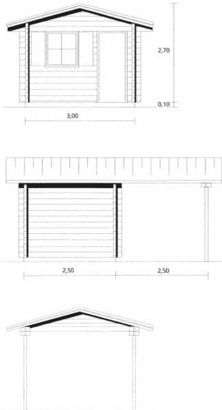
Chalethaus mit integrierem Vorbau
