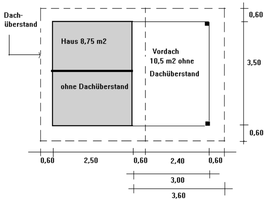
Detailzeichnung Pergola/Vordach im Familiengarten
